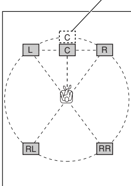
Klangbild des Mittellautsprechers
