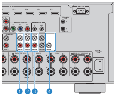
Gerät (Rückseite)
