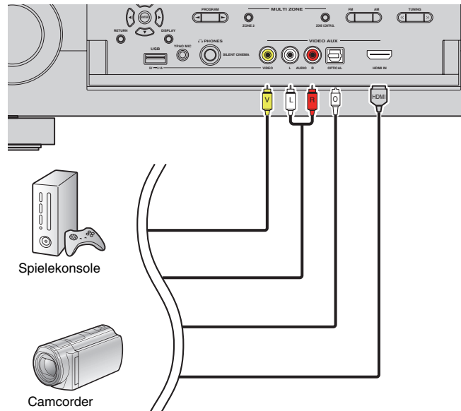
Gerät (Vorderseite)
