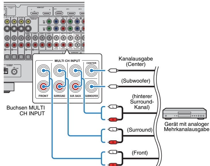
Gerät (Rückseite)
