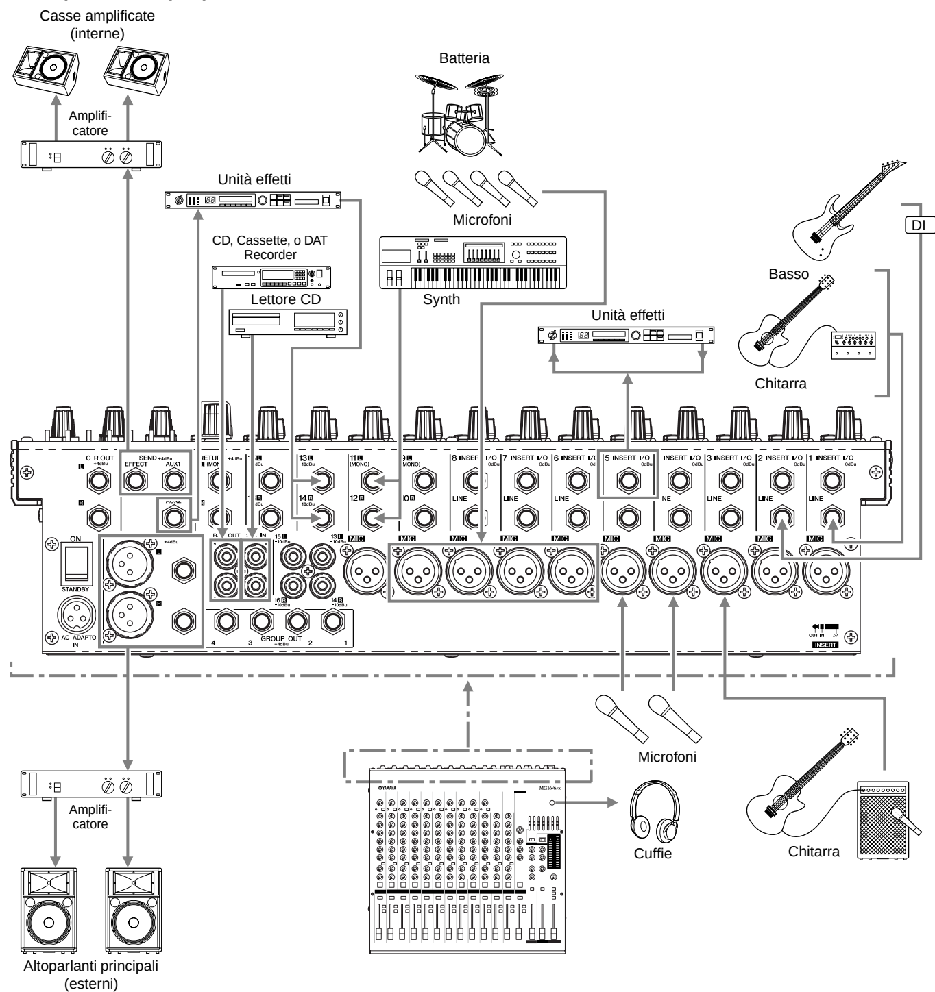
Esempio disposizione altoparlanti
