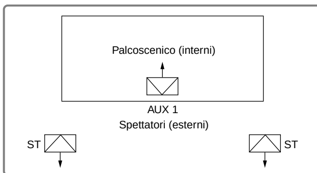
Esempio disposizione altoparlanti
