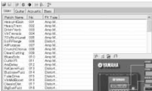
Archivfenster
