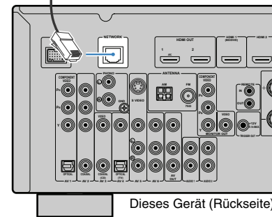
Netzwerk-kabel
