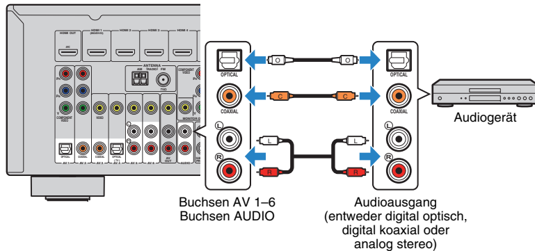
Gerät (Rückseite)
