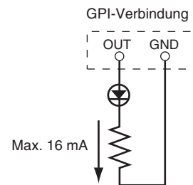
Beispiel: LED-Anzeigen externer Geräte vom DME Satellite aus aufleuchten lassen
