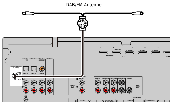
Gerät (Rückseite)
