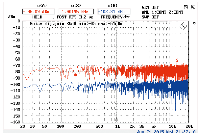
Störspektrum am Ausgang in dBu bei max. (rot) und min. (blau) Preamp Gain, gemessen am analogen Ausgang in dBu mit +20 dB dig. Gain (Abb. 5)
