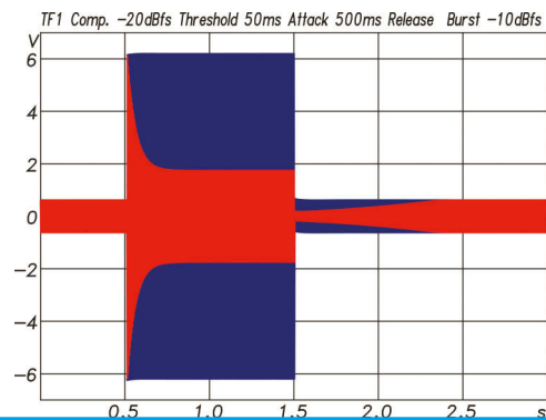
Kompressor Reaktion auf einen Sinusburst bei 50 ms Attack und 500 ms Release für einen Threshold-Wert -20 dBfs (Abb. 20)
