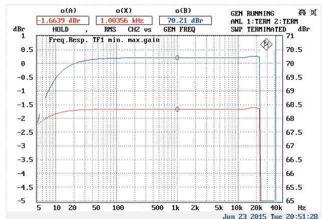
Frequenzgang über alles vom analogen Eingang zum analogen Ausgang gemessen bei min. Gain von -6 dB (rot) und bei max. Gain von +66 dB (blau) (Abb. 7)
