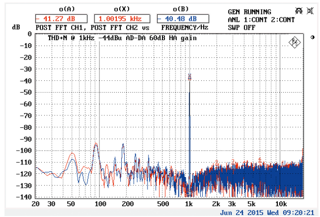
Klirrspektrum bei 60 dB Gain und -44 dBu Eingangspegel (Abb. 11)
