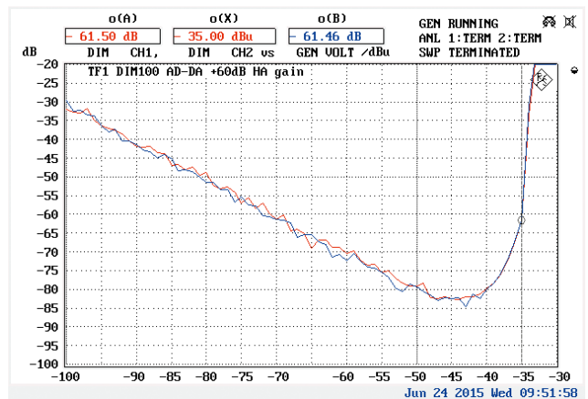
DIM Transiente Intermodulationsverzerrungen bei maximalem Gain (Abb. 13)
