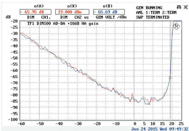
DIM Transiente Intermodulationsverzerrungen bei minimalem Gain (Abb. 12)
