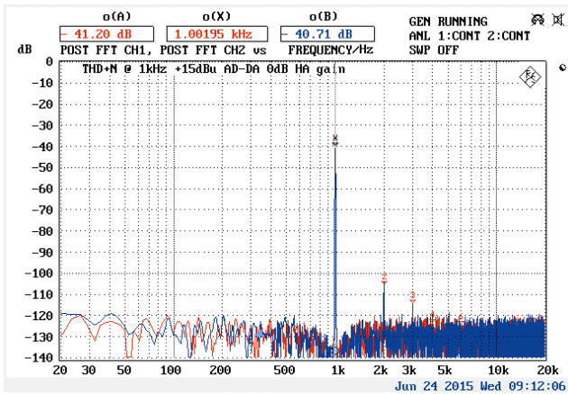
Klirrspektrum des TF1 bei 0 dB Gain und +15 dBu Eingangspegel (Abb. 10)
