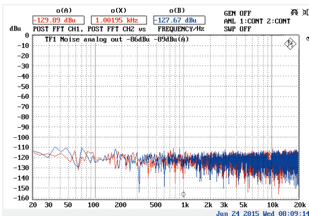
Störspektrum am analogen Ausgang bei zugezogenem Masterfader mit einem Gesamtpegel von -86 dBu lin. bew. und -89 dBu A-bew. Die maximale Ausgangsspannung beträgt +25 dBu. (Abb. 6)
