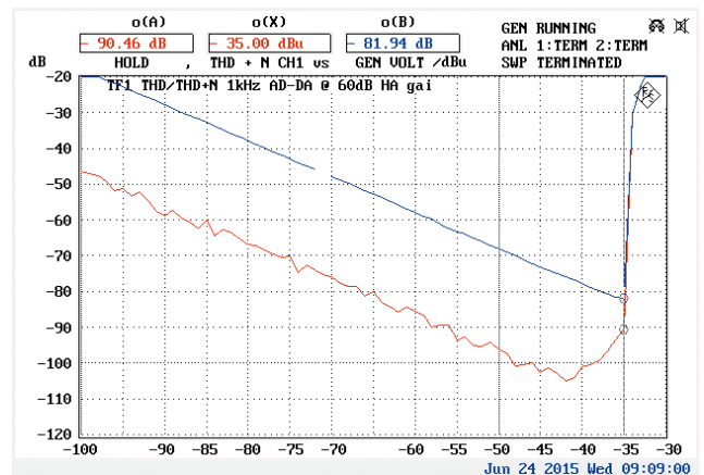
Gain von +60 dB THD (rot) und THD+N (blau), die Clipgrenze liegt dann bei -35 dBu Eingangspegel (Abb. 9)
