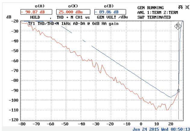
Preamp Gain 0 dB THD (rot) und THD+N (blau), die Clipgrenze liegt dann bei +25 dBu Eingangspegel (Abb. 8)
